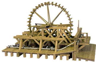
(Ill 3) Maquette de la machine de Modave (château de Modave)
